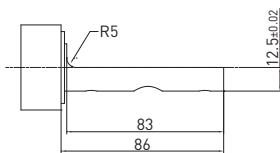
Stangeausführung 1
