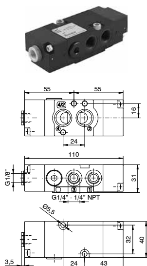
M51C.42.00.18 Peso 240 g
