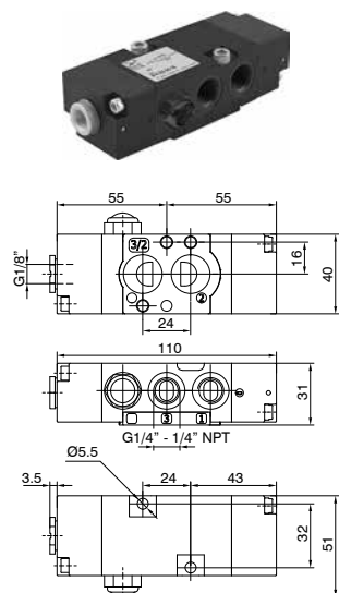
M51C.32.00.19C Peso 240 g
