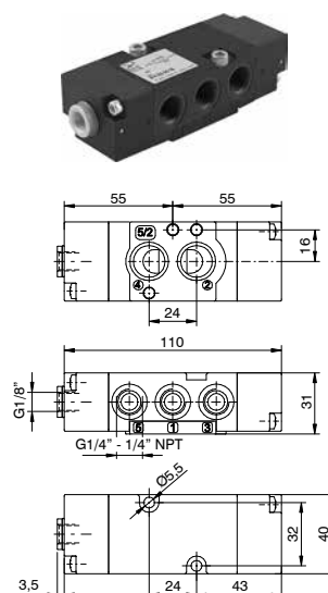
M51C.52.00.18 Peso 235 g
