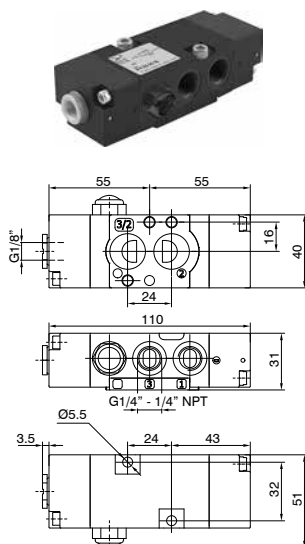
M51C.32.00.16 Peso 240 g
