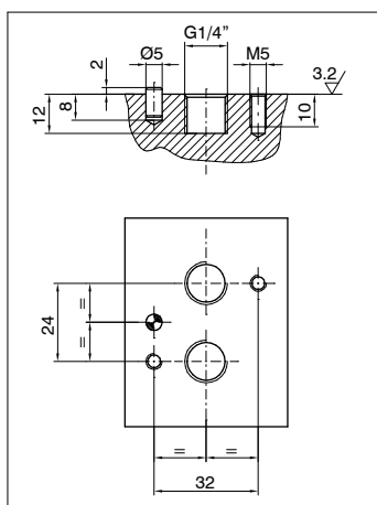
Dimensioni piano di posa NAMUR: secondo direttiva (VDI/VDE 3847 luglio 03)
