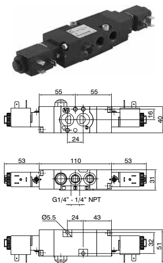
M51C.32.00.35.VC Peso 410 g
