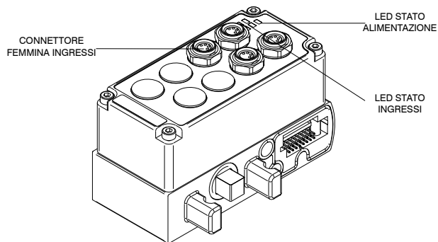
Connettore M8 4P Femmina
