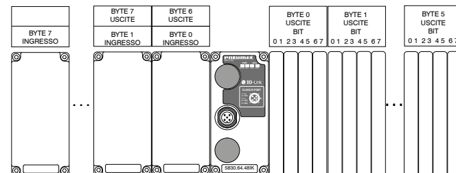
Esempio distribuzione dati di ingresso e di uscita con Interfaccia IO-Link 5830.64.48IK
