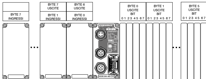
Esempio distribuzione dati di ingresso e di uscita con Interfaccia CANopen 5530.64.48CO
