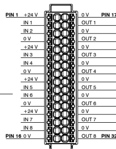
Morsettiere 32 pin
