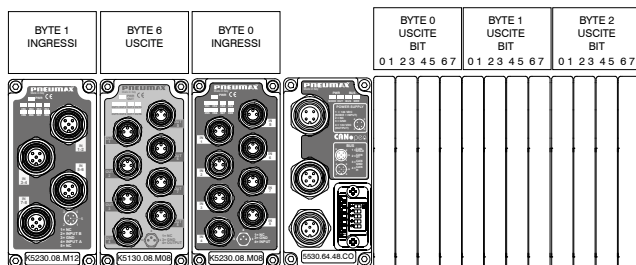
Esempio distribuzione dati di ingresso e di uscita con Interfaccia CANopen 5530.64.48CO
