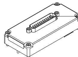
CONNETTORE SUB D 25 POLI
