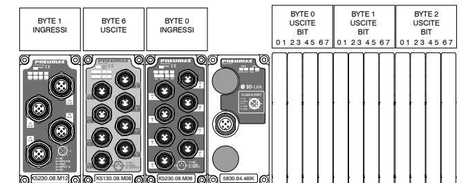
Esempio distribuzione dati di ingresso e di uscita con Interfaccia IO-Link 5830.64.48IK
