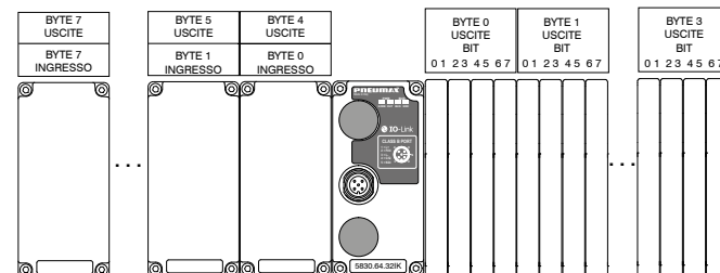
Distribuzione dati di ingresso e di uscita con Interfaccia IO-Link 5830.64.48IK
