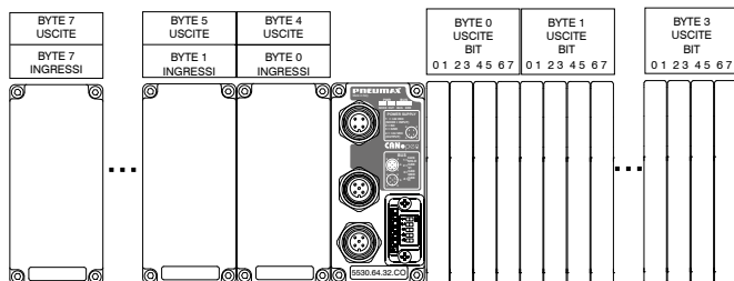
Distribuzione dati di ingresso e di uscita con Interfaccia CANopen 5530.64.48CO
