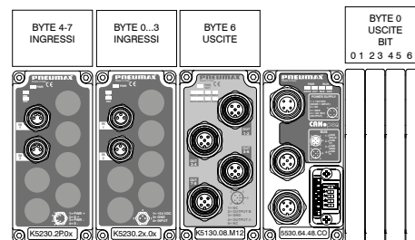
Esempio distribuzione dati di ingresso e di uscita con Interfaccia CANopen 5530.64.48CO
