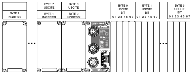
Esempio distribuzione dati di ingresso e di uscita con Interfaccia CANopen K5530.64.48CO
