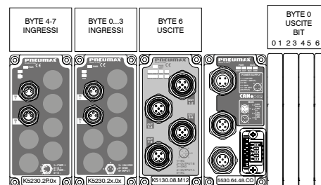
Esempio distribuzione dati di ingresso e di uscita con Interfaccia CANopen K5530.64.48CO
