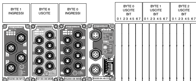
Esempio distribuzione dati di ingresso e di uscita con Interfaccia CANopen K5530.64.48CO
