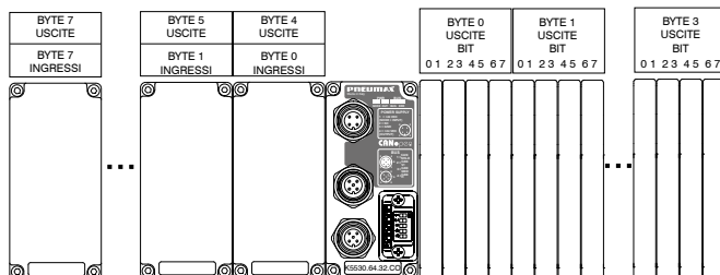
Distribuzione dati di ingresso e di uscita con Interfaccia CANopen K5530.64.48CO
